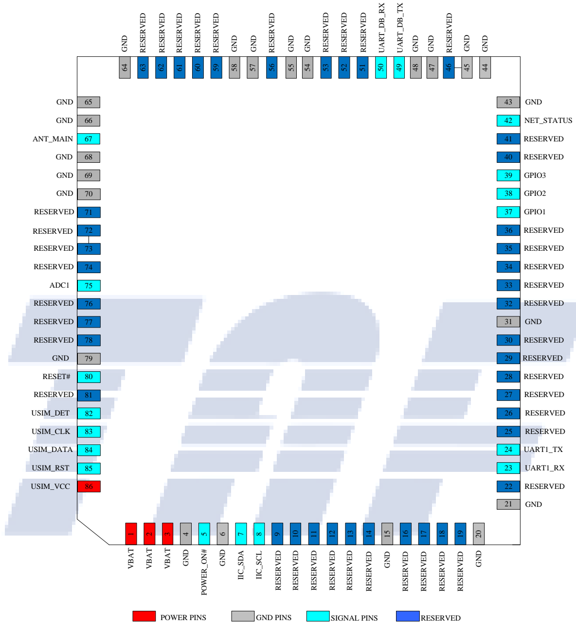
图1 管脚示意图(俯视图)
